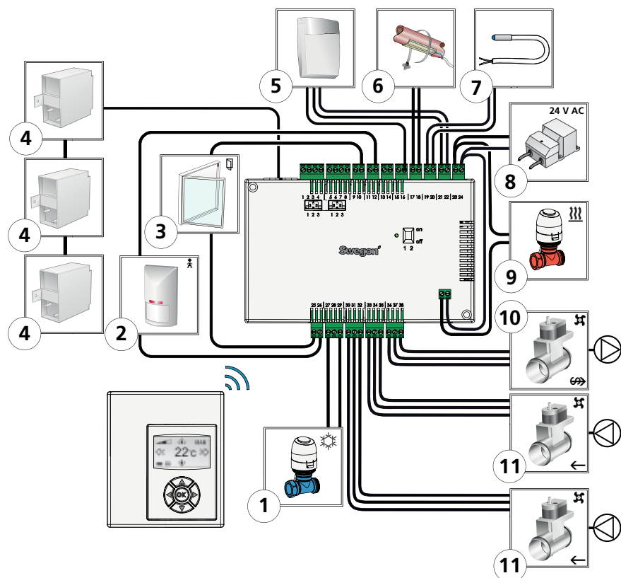
Figur 3. Översikt över enheter W4.2 (Konferens).
