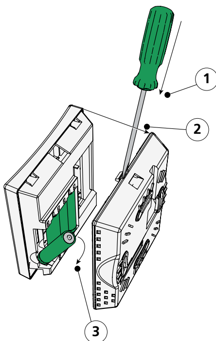
Figur 5. Montering av batterier i rumsenhet.
