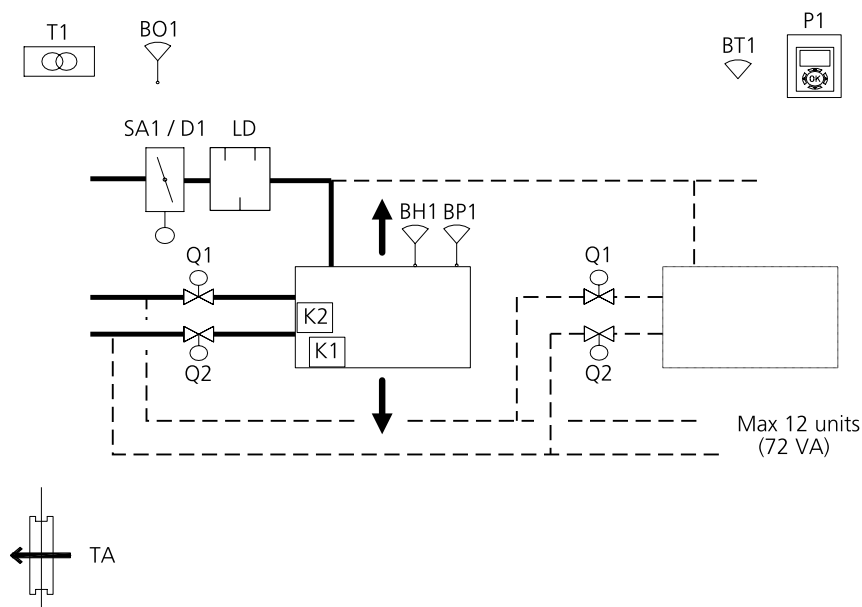
Figur 6. Exempel på installation med CONDUCTOR W4.1.
