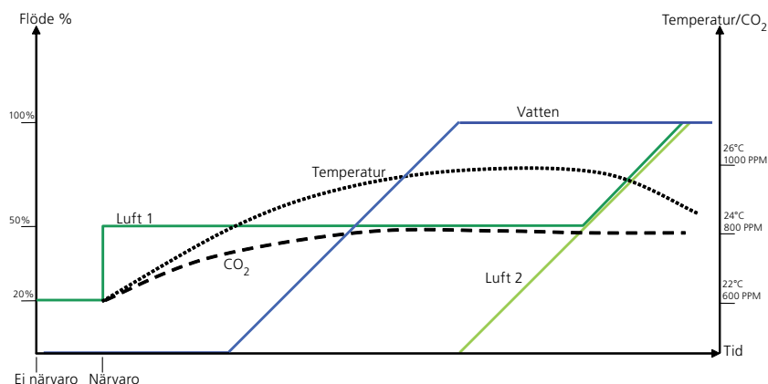
Figur 8. Exempel på diagram över sekvensen vatten-luft med temperaturkontroll. OBS! Luft 2 gäller endast W4.2
