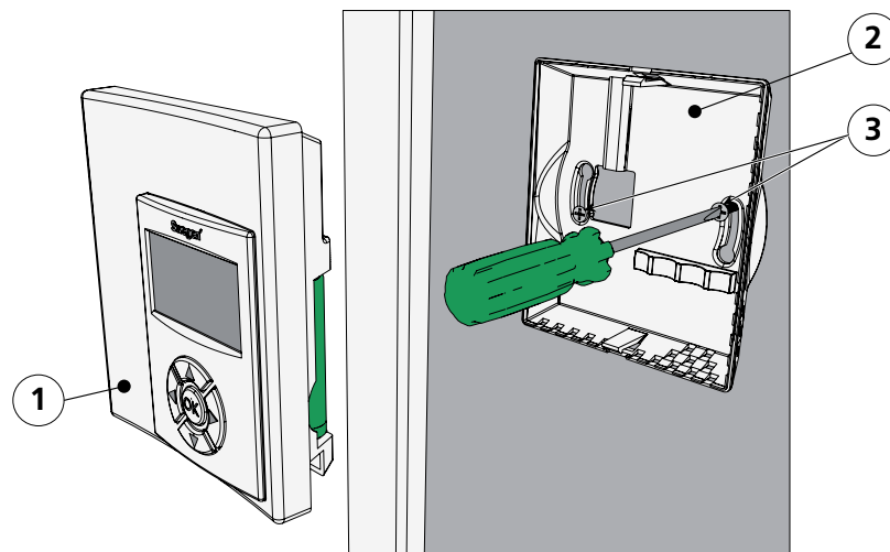
Figur 7. Montering av rumsenhet.
