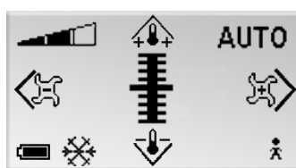
Figur 5. Huvudvyn.
