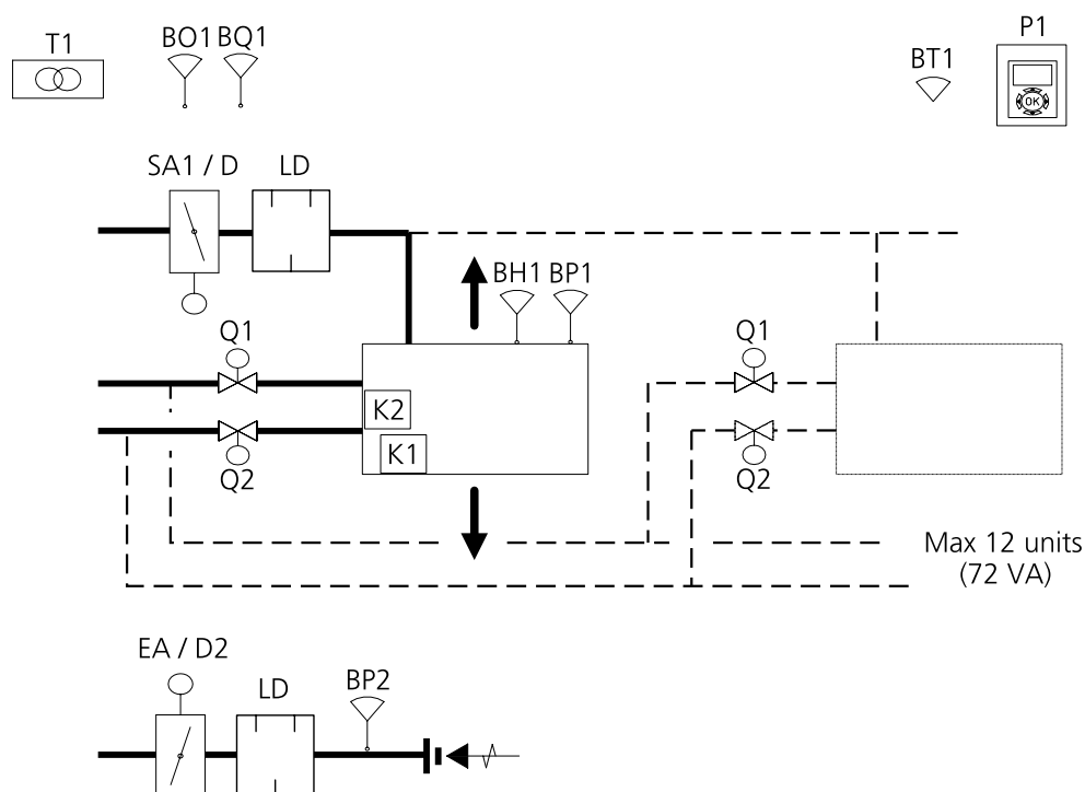
Figur 5. Exempel på installation med CONDUCTOR W4.1.
