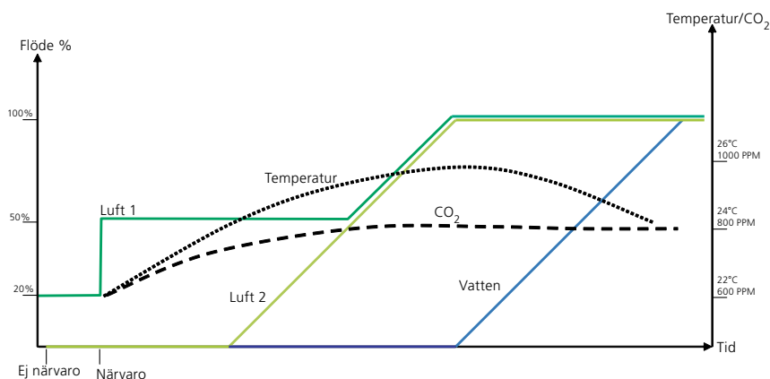
Figur 7. Exempel på diagram över sekvensen luft-vatten med temperaturkontroll. OBS! Luft 2 gäller endast W4.2
