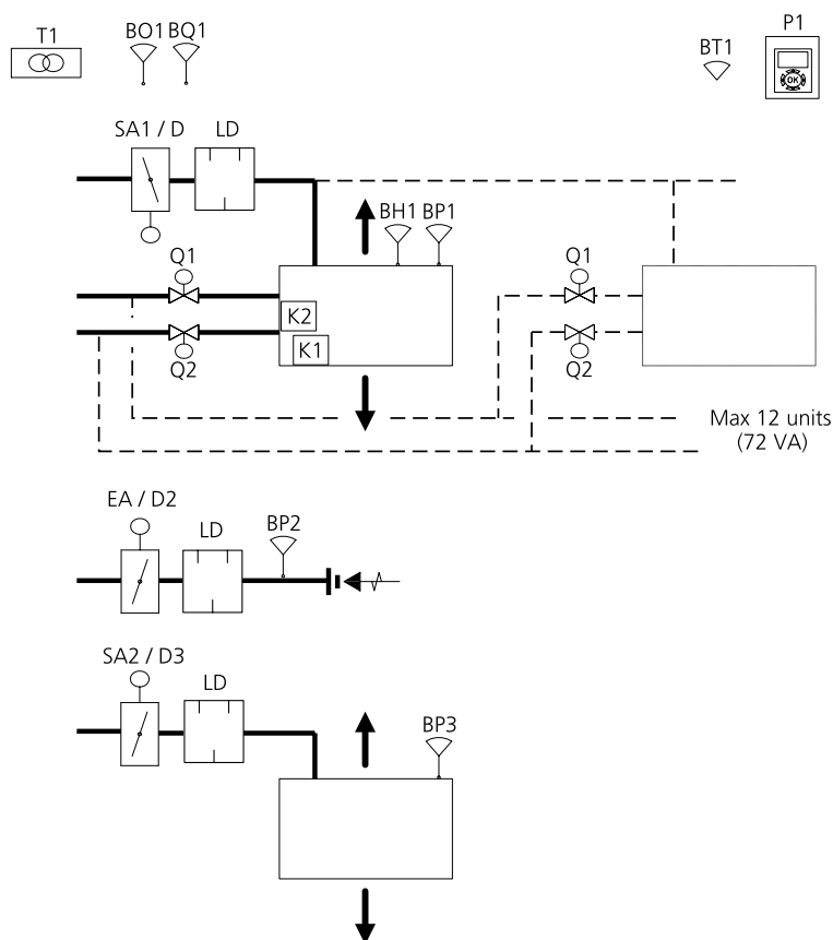
Figur 4. Exempel på installation med CONDUCTOR W4.2.
