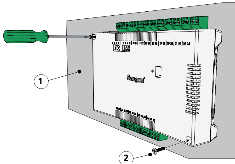
Figur 2. Montering av regulatören.
