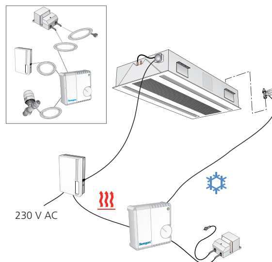
Figure 3. Connexion sur le bornier à vis pour épingle électrique
