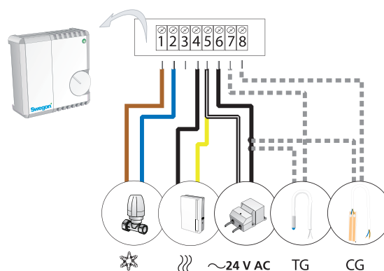
Figure 19. Connexion au bornier à vis du régulateur LUNA RE-S pour chauffage électrique
