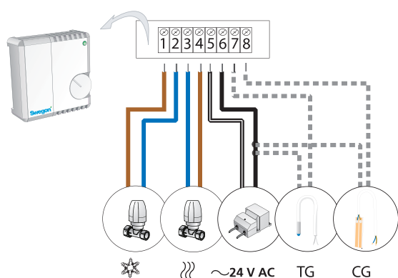
Figure 17. Raccordement sur la réglette du régulateur LUNA RE-S
