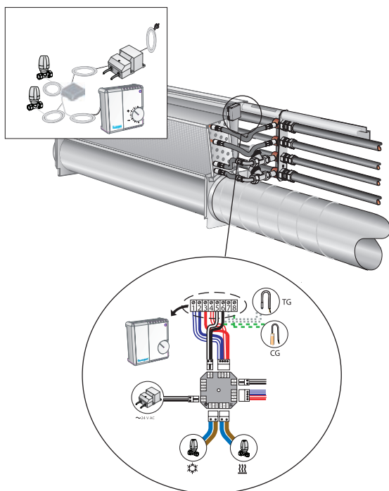
Figure 1. Montage en série avec carte de connexion et câbles préfabriqués.
