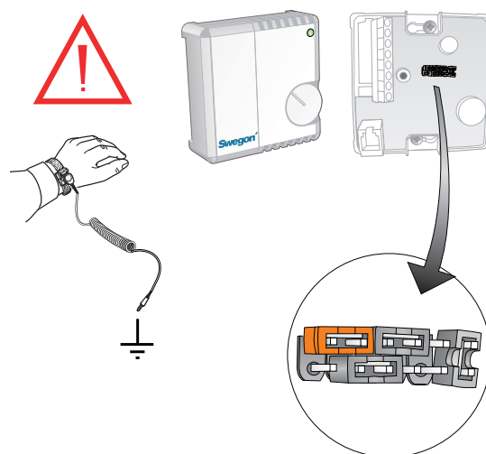
Figure 20. Repositionnement du cavalier pour chauffage électrique
