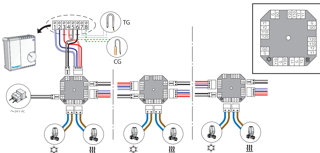
Figure 18. Raccordement en série de plusieurs LUNA KK associés au LUNA RE-1
