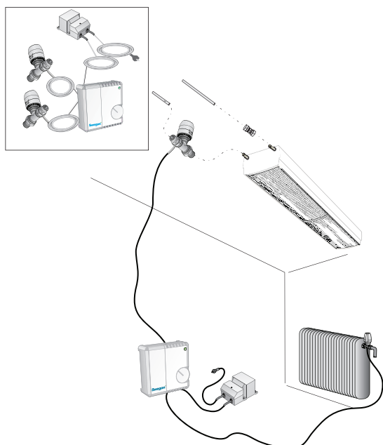
Figure 2. Raccordement sur la réglette du régulateur.
