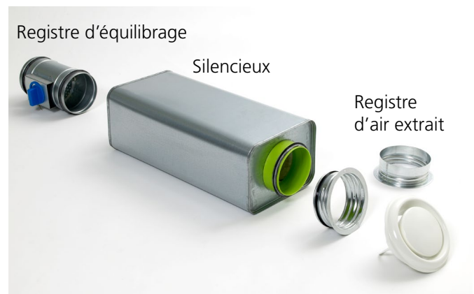
Figure 18. Kit d'air extrait - PARAGON T-EAK-CAV
