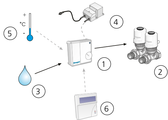
Figure 14. Système de régulation LUNA installé en usine
