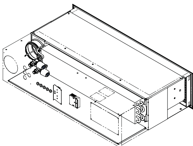
Figure 36. PARAGON Wall avec borniers de câblage LUNA montés en usine, vanne VDN215 et servomoteur ACTUATORb 24V NC.
