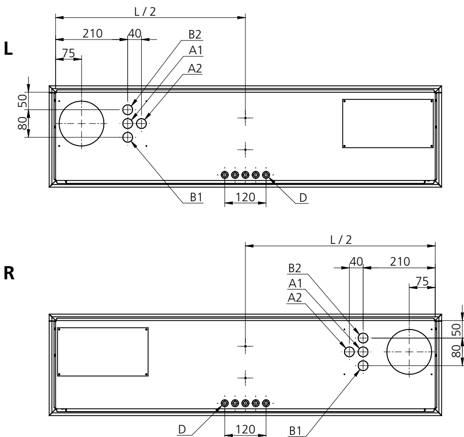
Figure 24. Vue de l'arrière, connexions R = modèle côté droit, L = modèle côté gauche
