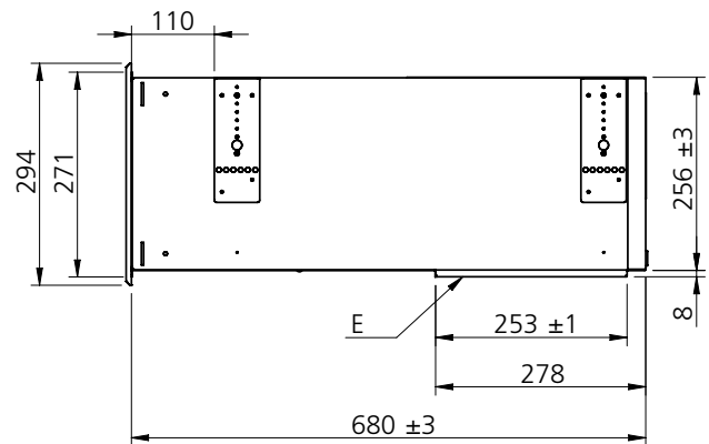
Figure 22. Vue du panneau d'extrémité
