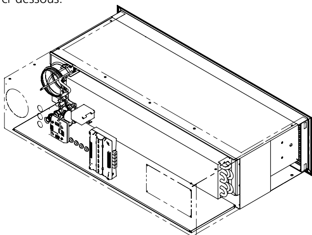
Figure 35. PARAGON Wall avec régulateur Conductor W4.1 monté en usine, comprenant un thermostat RU, une sonde de pression, une vanne VDN215 et un servomoteur ACTUATORb 24V NC de refroidissement et de chauffage.
