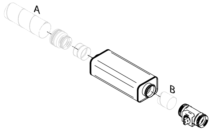
Figure 28. Kit d'air introduit, PARAGON T-SAK-CAV-100 Conduits spiralés taille 100 et manchons de jonction non compris. Conduit spiralé A: Longueur min.: 330 mm Conduit spiralé B: Longueur min.: 70 mm
