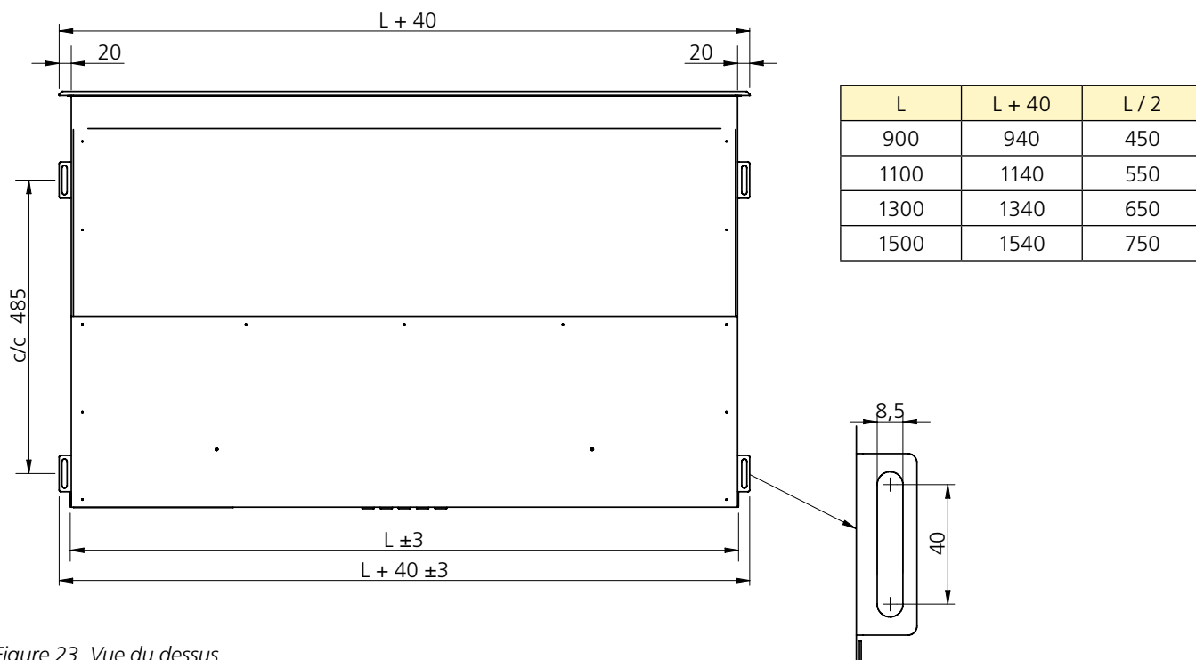
Figure 23. Vue du dessus
