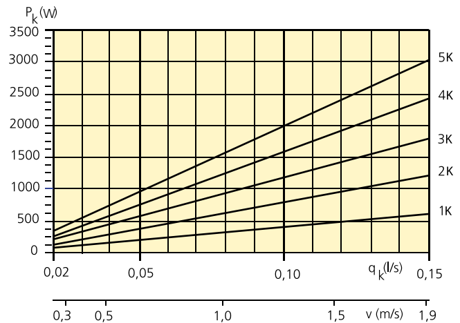
Diagramme 2. Débit d'eau – correction de capacité
