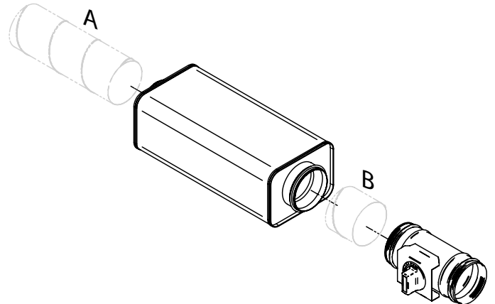
Figure 28. Kit d'air introduit, PARAGON T-SAK-CAV-125 Conduits spiralés non compris. Conduit spiralé A: Longueur min.: 330 mm Conduit spiralé B: Longueur min.: 70 mm
