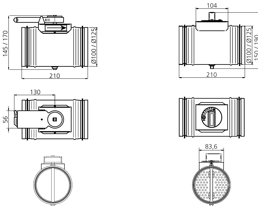
Figure 33. Cotes, registre motorisé. Inclus dans PARAGON T-SAK-CAV et PARAGON T-EAK-CAV
