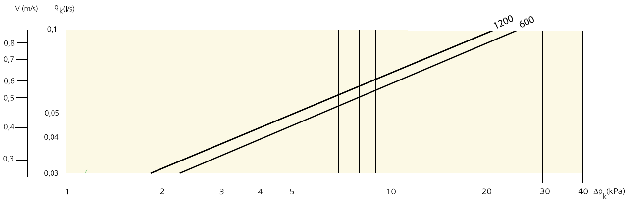
Diagramm 4. Druckabfall – Wasservolumenstrom Kühlung
