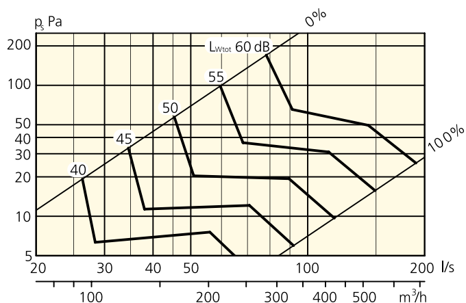
Diagramm 8. Einstellbereich, Klappe CRPc 9-160
