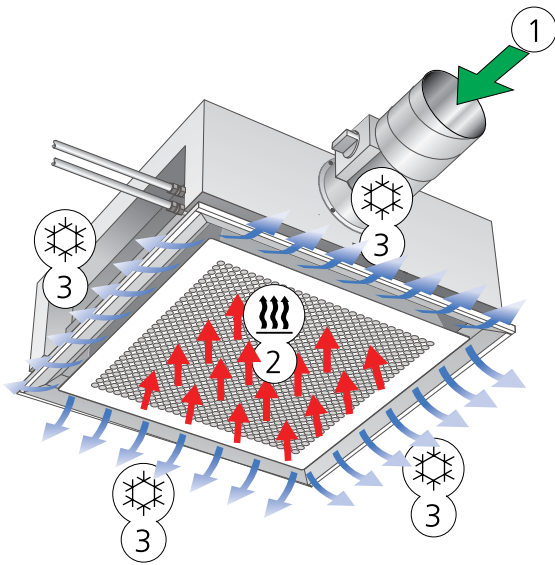
Abbildung 1. Variante A: Kühl- und Zulufffunktion 1 = Primärluft 2 = Induzierte Raumluft 3 = Primärluft gemischt mit gekühlter Raumluft
