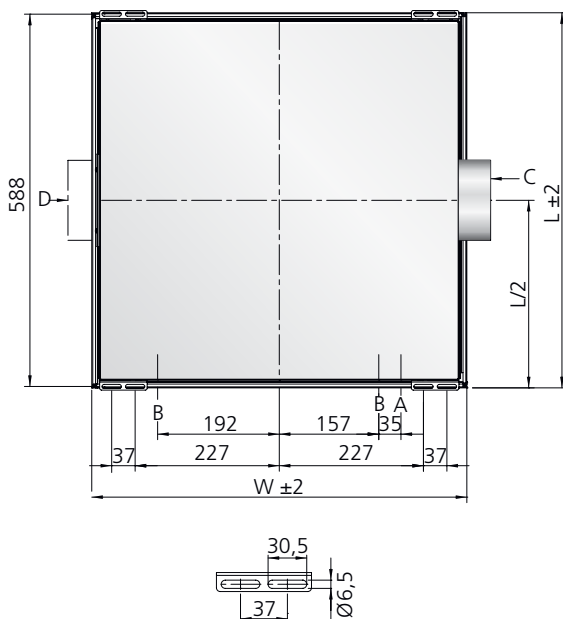
Abbildung 26. Parasol 600, Ansicht von oben A = Zu- und Ablauf Kühlwasser Ø12 x 1,0 mm (Cu) B = Zu- und Ablauf Warmwasser Ø12 x 1,0 mm (Cu) C = Anschlussstutzen für die Primärluft Ø125 mm D = Schloss über alternativem Luftanschluss
