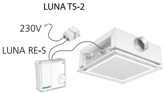
Abbildung 14. Typinstallation, wassergebundene Kühlung und Heizung
