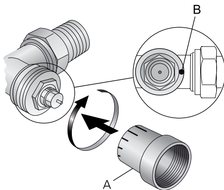
Abbildung 16. Einstellung des k_v -Werts. A = Schutzabdeckung, drehbar 180° B = Markierung an der Ausflusseite der Ventile
