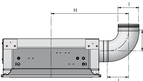
Abbildung 31. Anschluss mit Bogen, Vorderansicht Montiertes Verbindungsstück
