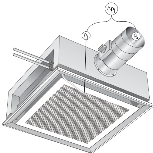
Abbildung 24. Druckverhalten Luft
