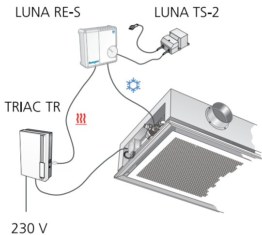
Abbildung 15. Wassergebundene Kühlung und Elektroheizung
