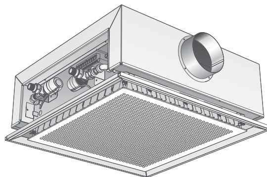
Abbildung 12. Werkseitig montierte Regelausrüstung LUNA (PARASOL b T-RK-LUNA)
