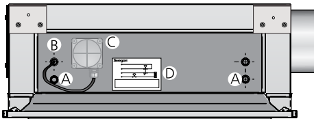
Abbildung 29. Parasol 1200 für Elektroheizung, Ansicht von vorne und Anschlüsse
