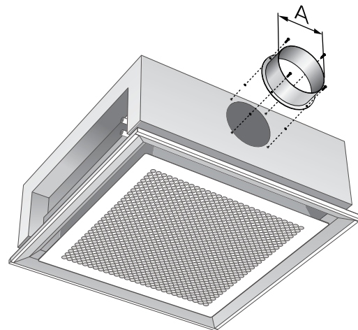
Abbildung 19. Luftanschlusstutzen
