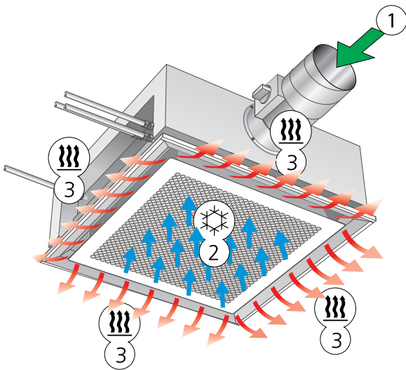
Abbildung 2. Variante B: Heizungs- und Zulufffunktion (auch mit integrierter Kühlfunktion) 1 = Primärluft 2 = Induzierte Raumluft 3 = Primärluft gemischt mit erwärmter Raumluft
