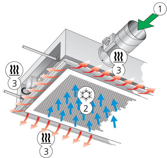
Abbildung 4. Variante X: Zuluff- und Heizungsfunktion mit Elektro- stäben (auch mit integrierter Kühlfunktion) 1 = Primärluft 2 = Induzierte Raumluft 3 = Primärluft gemischt mit erwärmter Raumluft
