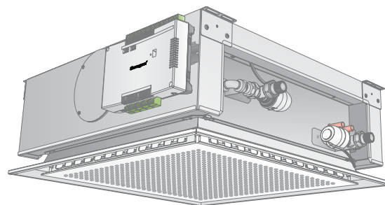
Abbildung 13. Werkseitig montierte Regelausrüstung CONDUCTOR (PARASOL b T-COND-XX)
