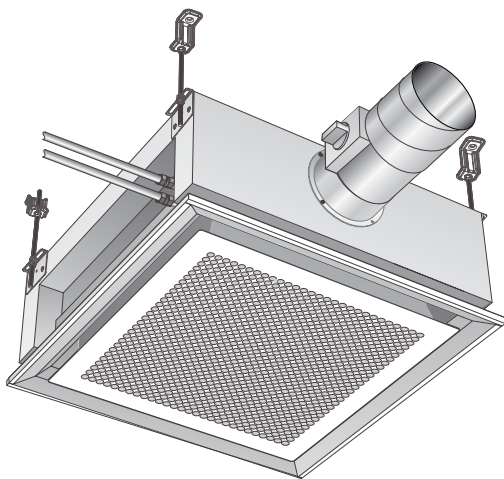
Abbildung 17. Aufhängen der Einmoduleinheit
