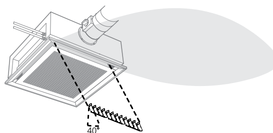
Abbildung 8. Einstellungsmöglichkeiten ADC II , X-shape
