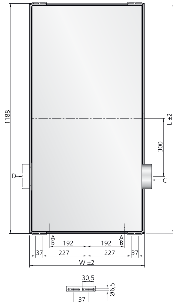
Abbildung 28. Parasol 1200, Ansicht von oben A = Zu- und Ablauf Kühlwasser Ø12 x 1,0 mm (Cu) B = Zu- und Ablauf Warmwasser Ø12 x 1,0 mm (Cu) C = Anschlussstutzen für die Primärluft Ø125 mm, PF= Ø160 mm D = Schloss über alternativem Luftanschluss
