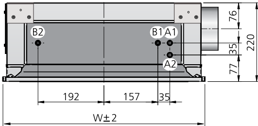
Abbildung 25. Parasol 600, Vorderansicht und Anschlüsse
