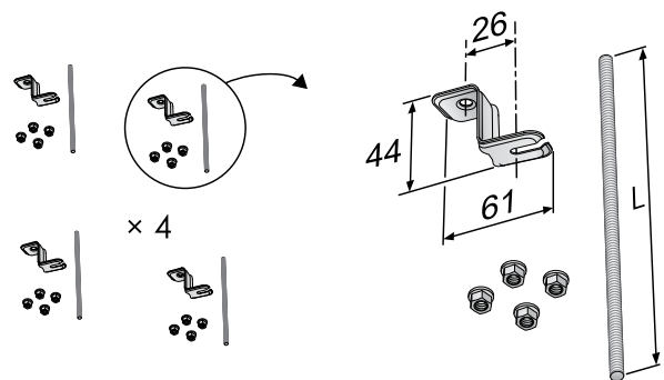
Abbildung 20. Montagestück SYST MS M6-1, Deckenbefestigung Gewindestange
