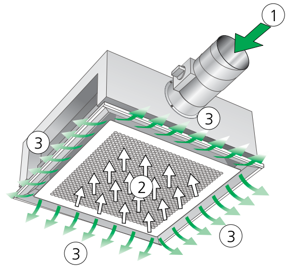
Abbildung 3. Variante C: Zulufffunktion 1 = Primärluft 2 = Induzierte Raumluft 3 = Primärluft gemischt mit Raumluft
