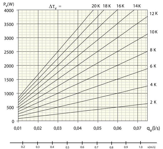
Diagramm 5. Volumenstrom Wasser - Heizkapazität
