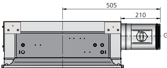
Abbildung 30. Anschluss mit Klappe, Vorderansicht E = Montierte Einstellklappe SYST CRPc 9-xxx
