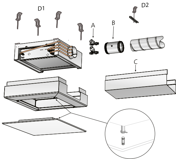
Abbildung 17. Anschlusskizze zur Aufhängung des Parasol EX und Gehäuse
