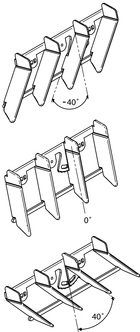
Abbildung 6. ADC II , Einstellungsbereich von -40° bis +40° in Schritten von 10°
