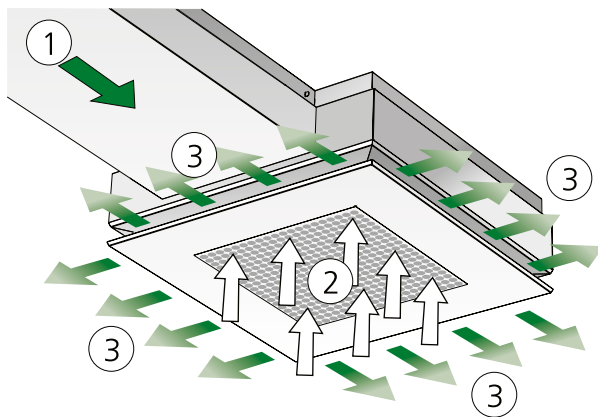
Abbildung 4. Variante C: Zulufffunktion
