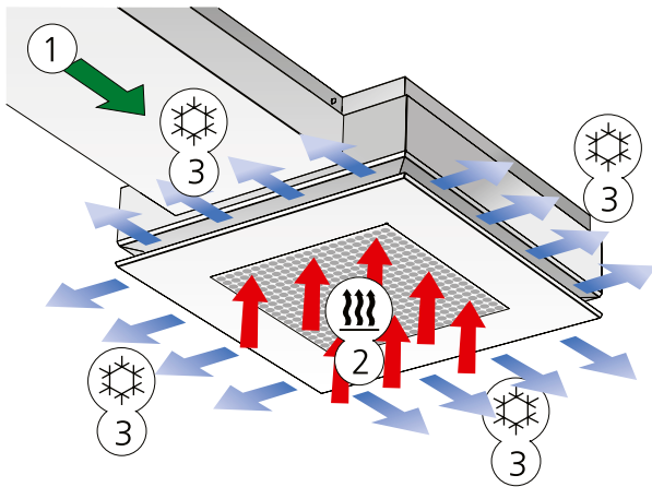
Abbildung 2. Variante A: Kühlfunktion
