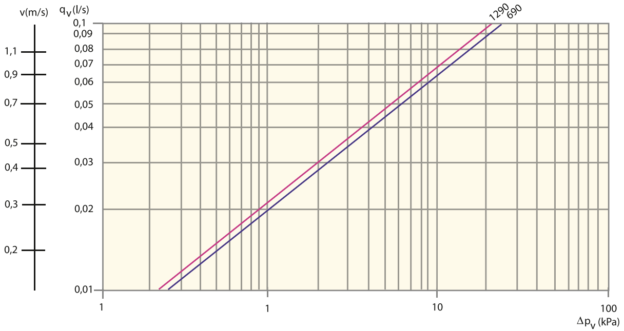
Diagramm 6. Druckabfall – Wasservolumenstrom Heizung
