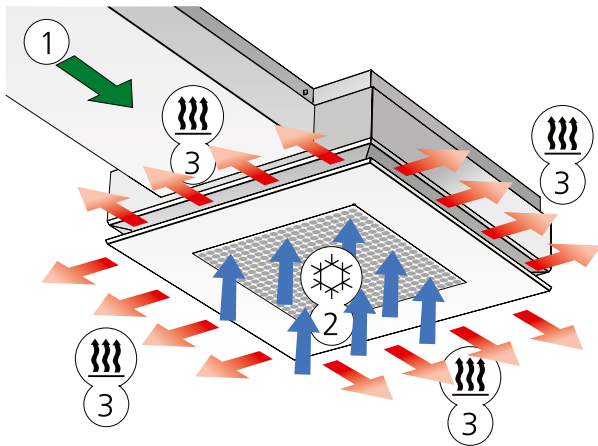
Abbildung 3. Variante B: Heizfunktion (inkl. Kühlfunktion)
