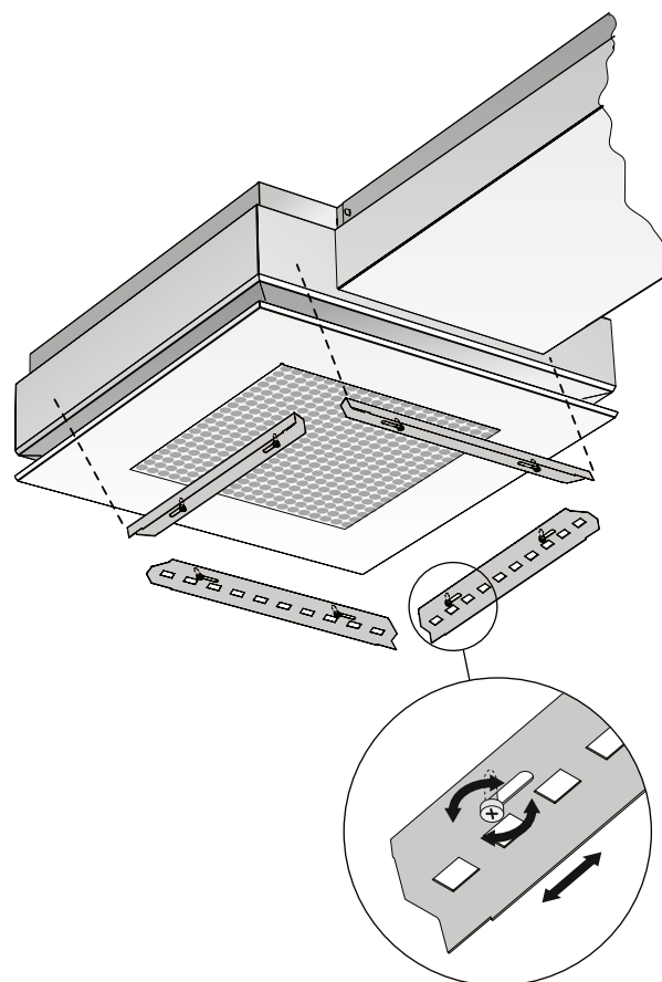
Abbildung 5. Düsenregulierung
