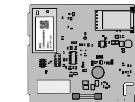
Figur 3. Kretskort.
