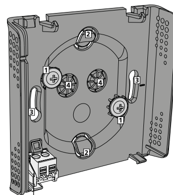
Inkoppling av strömförsörjning 24V AC/15-30V DC
