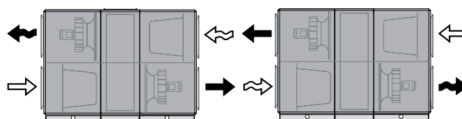
Fläktpos. 1 inställd som frånluft (högerinspektion)
