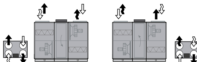
Fläktpos. 1 inställd som tilluft (vänsterinspektion)
