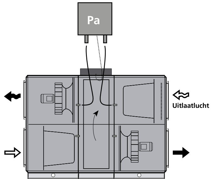
Aansluitprincipe voor de ontdooifunctie met aparte druksensor.
