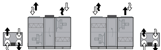
Puhaltimen sijainti 1 ase- tettu tuloilmaksi (tarkas- tuspouli vasemmalla)
