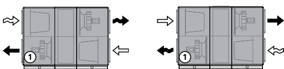
Zuluft unten (Links-Inspektion). Nicht RX Größe 004-008 in gemeinsamem Gehäuse.
