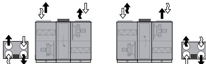
Ventilatorpos. 1 indstillet som tilluft (venstreinspektion)
