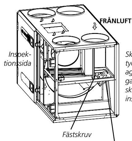
Injusteringsplåt
