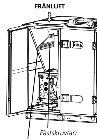
Injusteringsplåt
