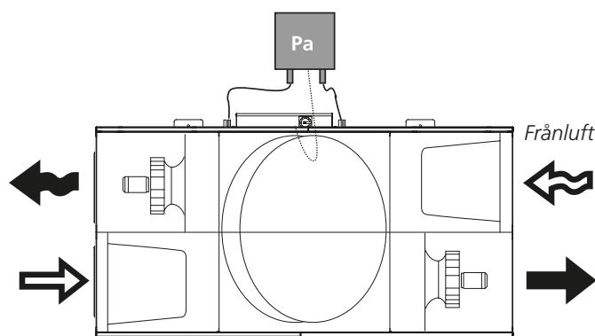
Princip för avfrostningsfunktion med separat tryckgivare.
