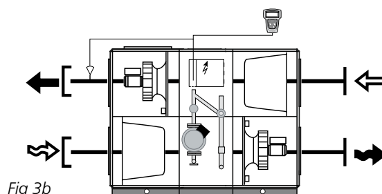
Vänsterutförande fläktplacering 1
