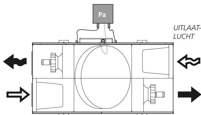
Principe voor ontdooien met separate druksensor.
