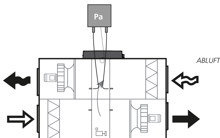
Prinzip der Enteisungsfunktion mit separatem Druckfühler.
