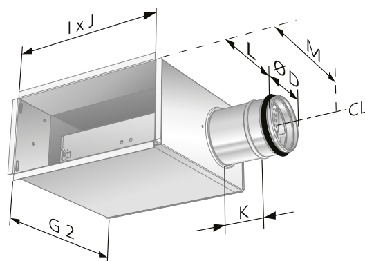
Figur 4. LOCKZONE W med anslutningslåda ALV.
