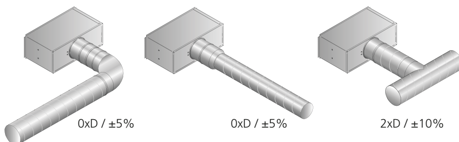
Figur 2. Monteringsalternativ, gäller för alla anslutningar (B, K)
