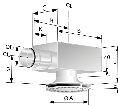
Kuva 4. CDK/CKP + ALS.
