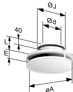
Kuva 3. CDK/CKP.
