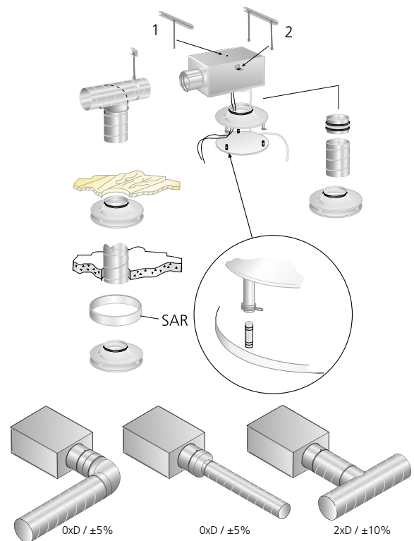
Kuva 2. Asennus.
