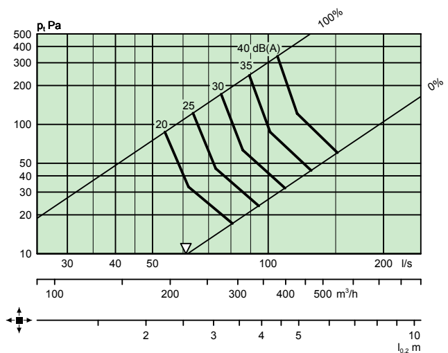
CKP 200 + ALS 160-200
