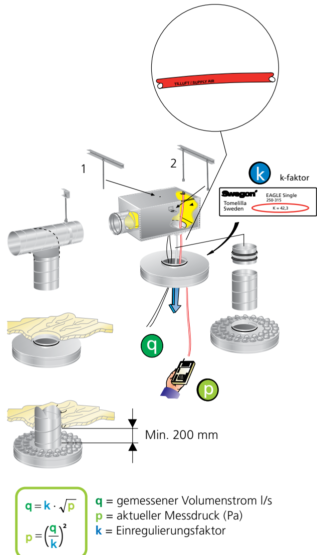
Abbildung 1. Montage Einregulierung.
