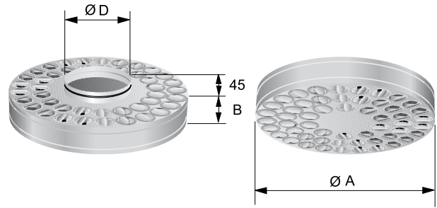
Abbildung 2. Luftauslass S/D.
