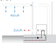
Technikraumgerät AirBlue PLT Funktionsschema
