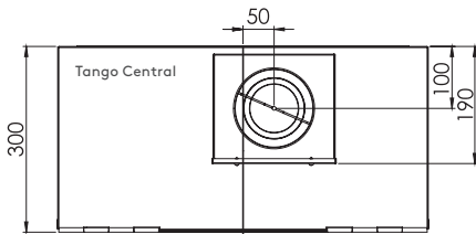
Tango Central ylänäkö CSB kuristinlaatikko vakiona
