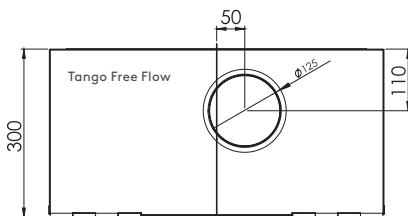
Tango Free Flow ylänäkö
