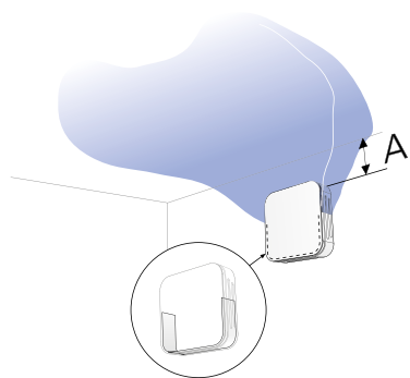
Abbildung 4: Einweg, Wandmontage
