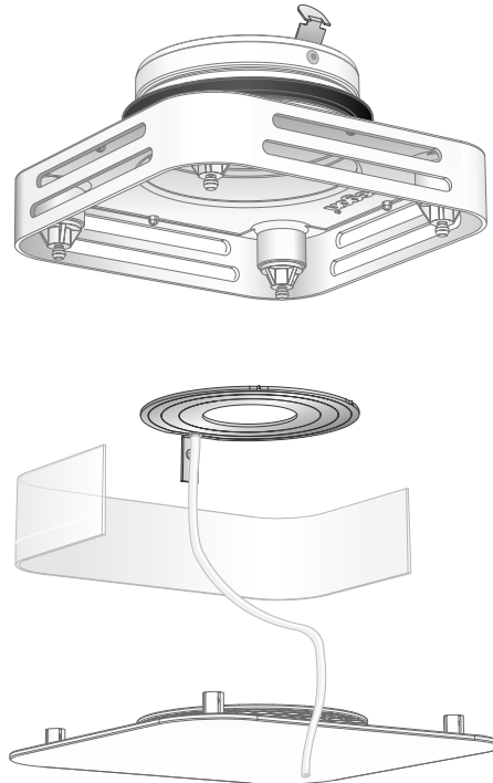
Abbildung 1: Montage, Einstückung
