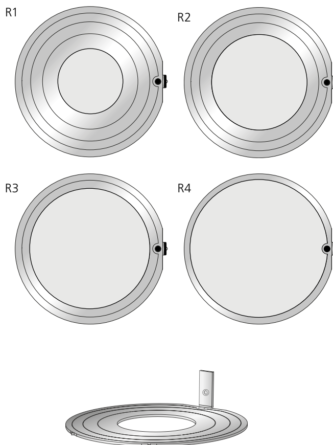
Abb. 5. Teilbare Einregulierungsscheibe. R1-4 zeigt verschiedene Einstellungsoptionen mit Messanschluss an der 3-Uhr-Position.
