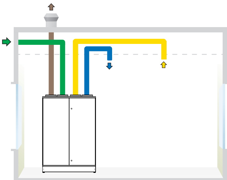
CASA W9 med golvsockel
