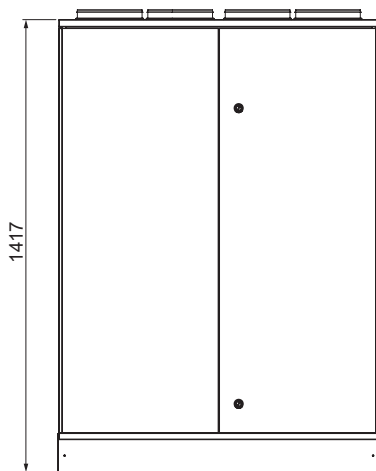
CASA W9 med golvsockel
