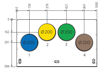
CASA W9 R, högerutförande
