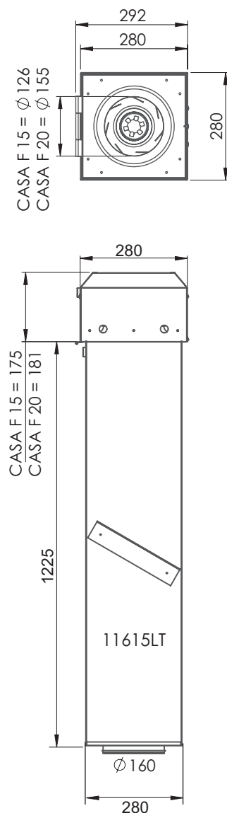
CASA F 15 & CASA F 20
