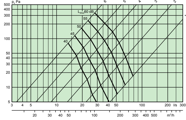
SIRI 125
