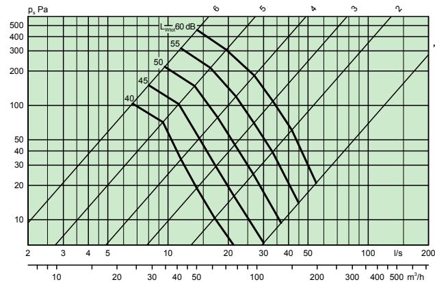
SIRI 100
