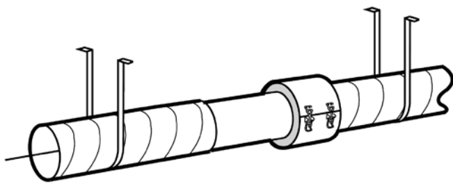
Figur 1. Montering. Fritt utrymme mellan kanaländar = Detaljens totallängd + 10 mm.
