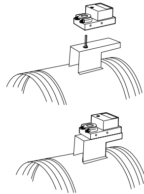
Kuva 3. Moottorin asennus, koko 100-400.
