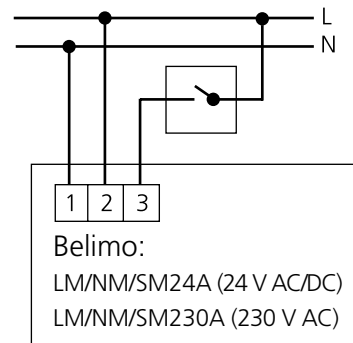
Kuva 8. KytKentäkaavio Belimo, 2-pistesäättö.
