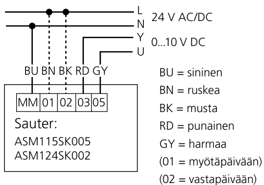
Kuva 7. KytKentäkaavio Sauter, 0-10 V vaihteleva/moduloiva säätö.
