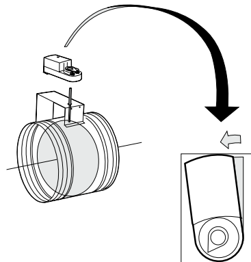
Kuva 4. Moottorin asennus CRT, koko 500 ja 630. Sulje pelti kokonaan. Sen jälkeen asenna moottori suoraan asentoon ja lukitse moottori akseliin. Kierrä moottoria 5° suljetusta asennosta ja lukitse sen jälkeen moottorin asento.
