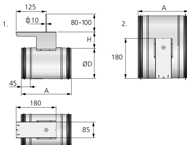
Kuva 11. CRT, mitat (mm).
