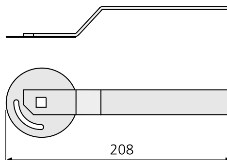
Kuva 12. Säätekahva CRTT-1, mitat (mm).
