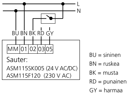
Kuva 5. KytKentäkaavio Sauter, 2-pistesäättö.
