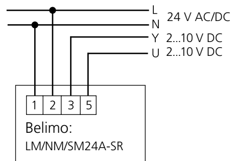
Kuva 10. KytKentäkaavio Belimo, 2-10 V vaihteleva/moduloiva säätö.
