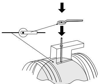
Kuva 2. Kahva asennus, CRTT-1
