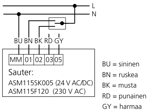
Kuva 6. KytKentäkaavio Sauter, 3-pistesäättö.
