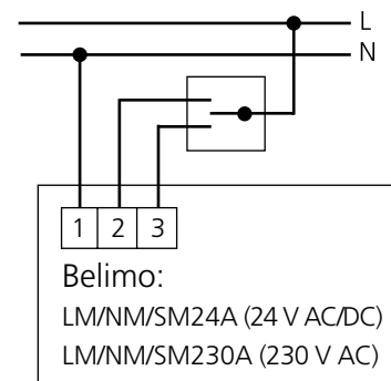
Kuva 9. KytKentäkaavio Belimo, 3-pistesäättö.
