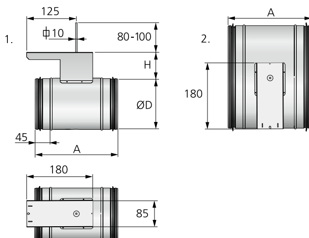
Figur 11. Mål CRT (mm).
