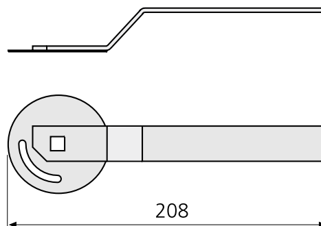
Figur 12. Mål, greb CRTT-1 (mm).
