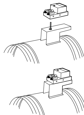
Figur 3. Montering motor, størrelse 100-400.
