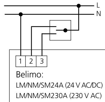
Figur 9. Tilslutningsdiagram Belimo, 3-punktsregulering.
