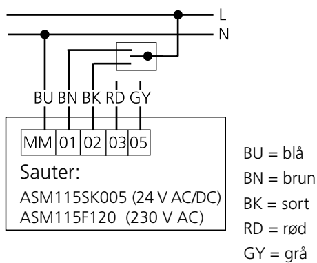
Figur 6. Tilslutningsdiagram Sauter, 3-punktsregulering.
