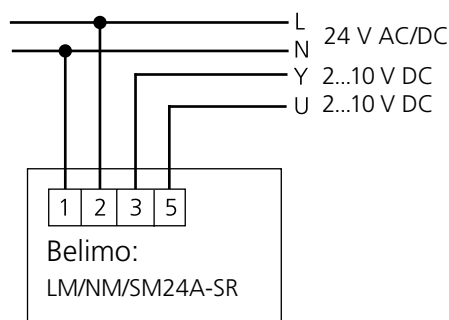
Figur 10. Tilslutningsdiagram Belimo, 2-10 V trinløs/module-rende regulering.
