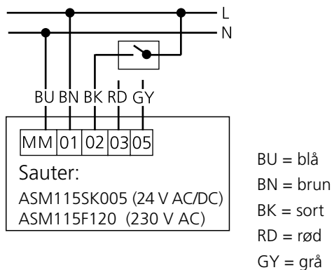
Figur 5. Tilslutningsdiagram Sauter, 2-punktsregulering.
