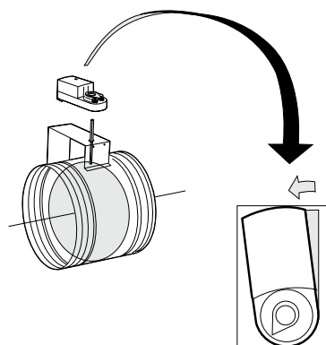
Figur 4. Montering motor CRT, størrelse 500 og 630. Luk spjældet helt. Monter derefter motoren helt lige, og lås motoren mod spjældakslen. Drej motoren 5° forbi lukket position, og lås motorens position.
