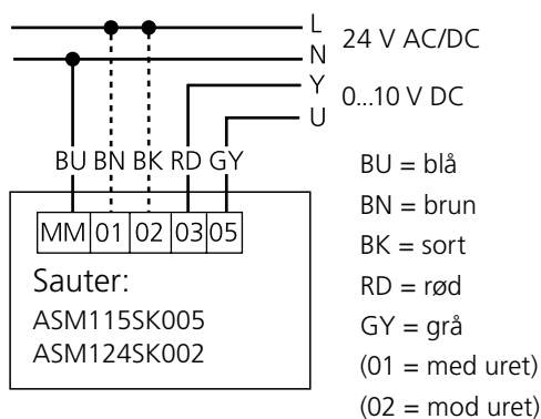
Figur 7. Tilslutningsdiagram Sauter, 0-10 V trinløs/modulerende regulering.
