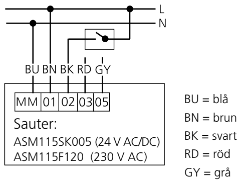
Figur 4. Kopplingsschema Sauter, 2-punktsreglering.
