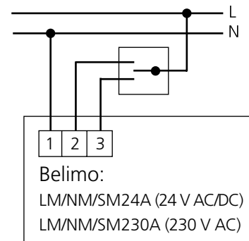
Figur 8. Kopplingsschema Belimo, 3-punktsreglering.
