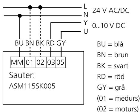
Figur 6. Kopplingsschema Sauter, 0-10 V steglös/modulerande reglering.
