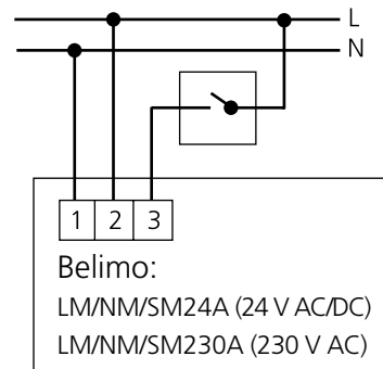
Figur 7. Kopplingsschema Belimo, 2-punktsreglering.
