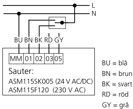
Figur 5. Kopplingsschema Sauter, 3-punktsreglering.
