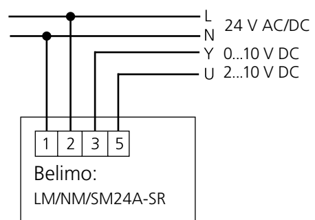
Figur 9. Kopplingsschema Belimo, 0-10 V steglös/modulerande reglering.
