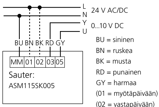
Kuva 6. KytKentäkaavio Sauter, 0-10 V vaihteleva/moduloiva säätö.
