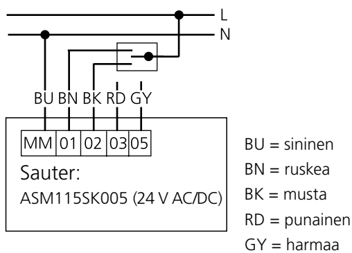
Kuva 5. KytKentäkaavio Sauter, 3-pistesäätö.
