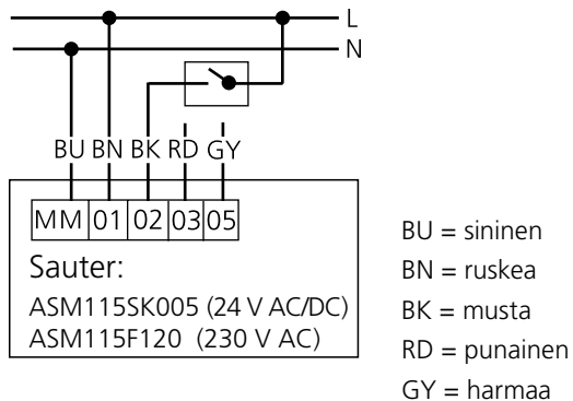
Kuva 4. KytKentäkaavio Sauter, 2-pistesäätö.
