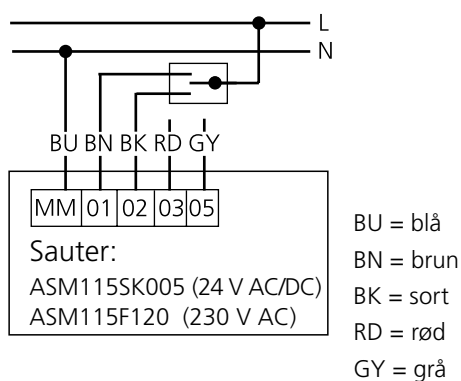
Figur 5. Tilslutningsdiagram Sauter, 3-punktsregulering.
