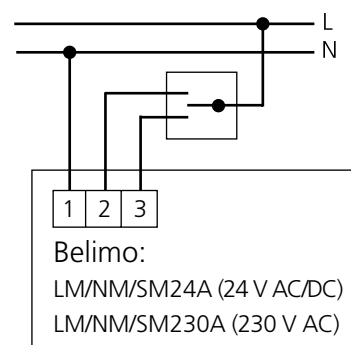
Figur 8. Tilslutningsdiagram Belimo, 3-punktsregulering.
