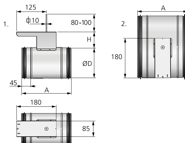
Figur 12. Mål (mm), CRP. 1. CRP-(100-400)-4 2. CRP-(500-630)-4
