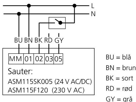
Figur 4. Tilslutningsdiagram Sauter, 2-punktsregulering.
