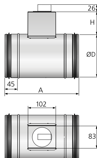
Figur 11. Mål (mm), CRP-xxx-1.
