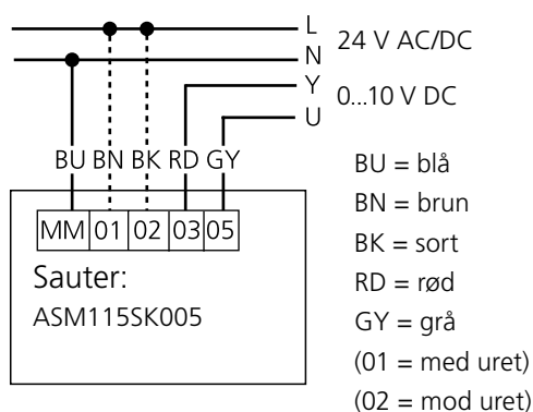
Figur 6. Tilslutningsdiagram Sauter, 0-10 V trinløs/modulerende regulering.
