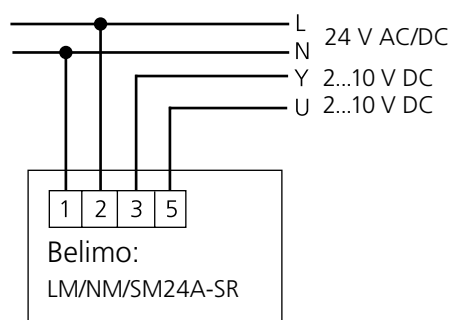
Figur 9. Tilslutningsdiagram Belimo, 0-10 V trinløs/modulerende regulering.
