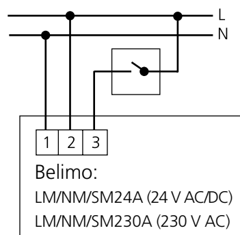
Figur 7. Tilslutningsdiagram Belimo, 2-punktsregulering.
