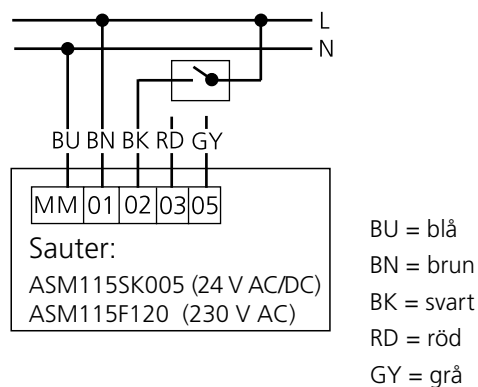
Figur 6. Kopplingsschema Sauter, 2-punktsreglering.
