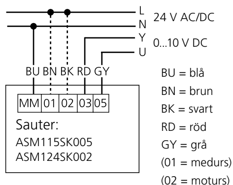
Figur 8. Kopplingsschema Sauter, 0-10 V steglös/modulerande reglering.
