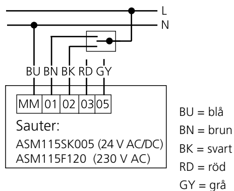
Figur 7. Kopplingsschema Sauter, 3-punktsreglering.
