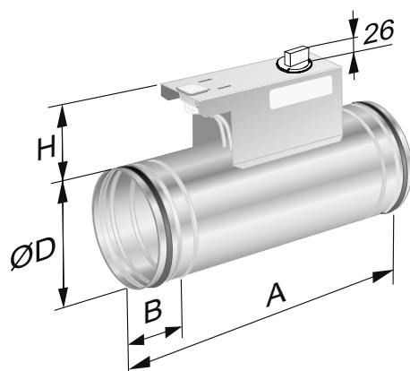
Figur 12. Mått (mm), CRM utan motor.
