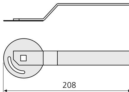
Figur 14. Mått (mm), vred CRTT-1.
