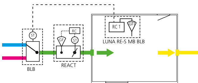
Figur 1. Funktionsbeskrivning av BLB för elektriskt regelsystem i kombination med REACT och LUNA RE-S MB BLB.
