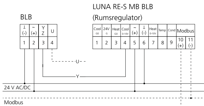
Figur 3. Kopplingsschema, BLB med elektrisk motor.
