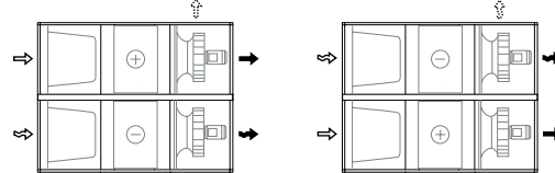
Fläktplacering 5, tilluft uppe
