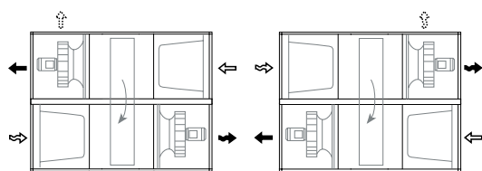
Tilluftsfläkt, vänster, uppe Tilluftsfläkt, vänster, nere Vänsterutförande
