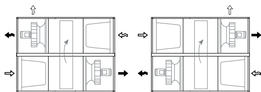
Tilluftsfläkt, höger, nere Tilluftsfläkt, höger, uppe Högerutförande
