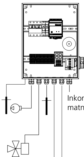
Apparatlåda 809535, rörkopplingsenhet (tillbehör, se separat installationsanvisning)
