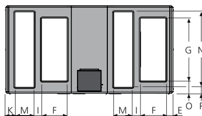
Vista dall'alto. Mostra i collegamenti canali dell'unità di trattamento aria per il ventilatore dell'aria di mandata con il lato destro in basso e sinistro in alto
