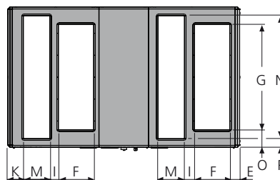
Vista dall'alto. Mostra i collegamenti canali dell'unità di trattamento aria per il ventilatore dell'aria di mandata con il lato destro in basso e sinistro in alto
