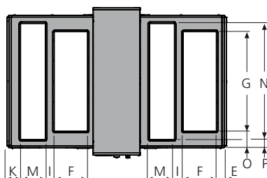
Vue du dessus. Montre les raccords de gaine de la centrale de traitement d'air pour le ventilateur d'air soufflé en bas à droite et en haut à gauche
