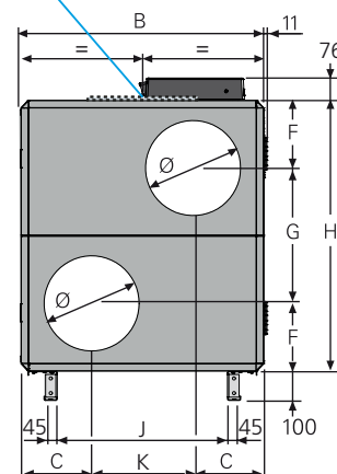
Sähköliitäntä
