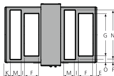
Näkymä ylhäältä. Kuvassa näkyvät koneen kanavaliitännät tuloilmapuhallinta varten oikealla alhaalla ja vasemmalla ylhäällä
