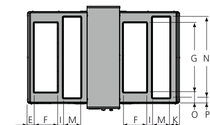
Näkymä ylhäältä. Kuvassa näkyvät koneen kanavaliitännät tuloilmapuhallinta varten oikealla ylhäällä ja vasemmalla alhaalla
