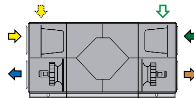
Vasenkätinen
