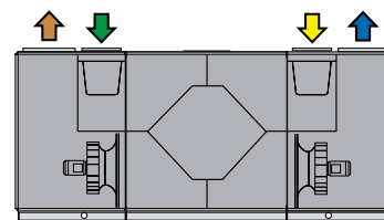
Oikeakätinen
