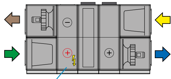
Batteria di riscaldamento elettrica posta in RX/HC (accessoria)
