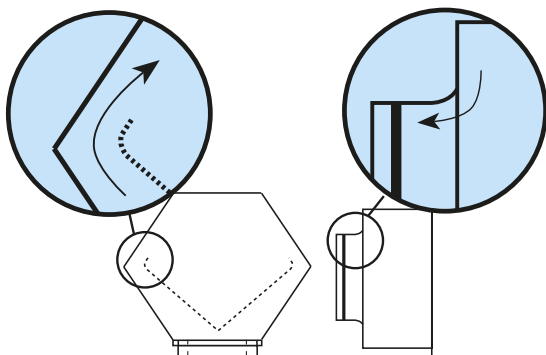
Réduction des pertes de pression grâce à des déflecteurs et prises d'air extrudées - voir accessoires Swegon pour centrale GOLD
