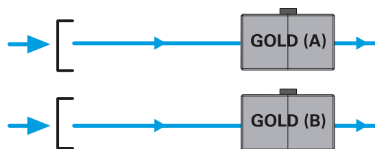
Chaque centrale GOLD doit être dotée d'un conduit d'air extérieur (et d'un capot ou conduit d'air extrait).
