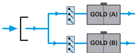
Si l'on souhaite utiliser un conduit d'air extérieur commun, le conduit correspondant de chaque centrale GOLD doit être doté d'un clapet de non-retour ou d'un registre à moteur (même chose dans le cas d'un capot ou conduit d'air extrait commun).
