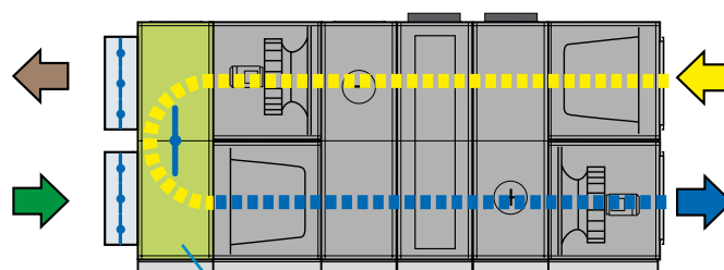
Umluftsektion RX/HC (Zubehör)
