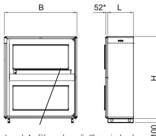
Umluftsektion RX/HC (Zubehör)
