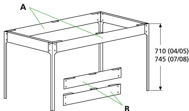
Stativ für GOLD RX/SD, Größe 004/005 und 007/008.
