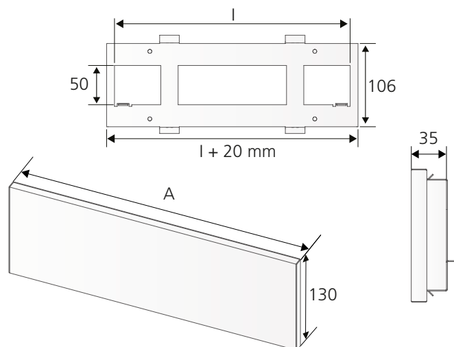
Kuva 3. ORTO, mitat.
