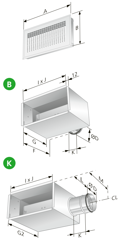
Kuva 4. Mitat, LOCKZONE Wall ja ALV-liitäntälaatikko.
