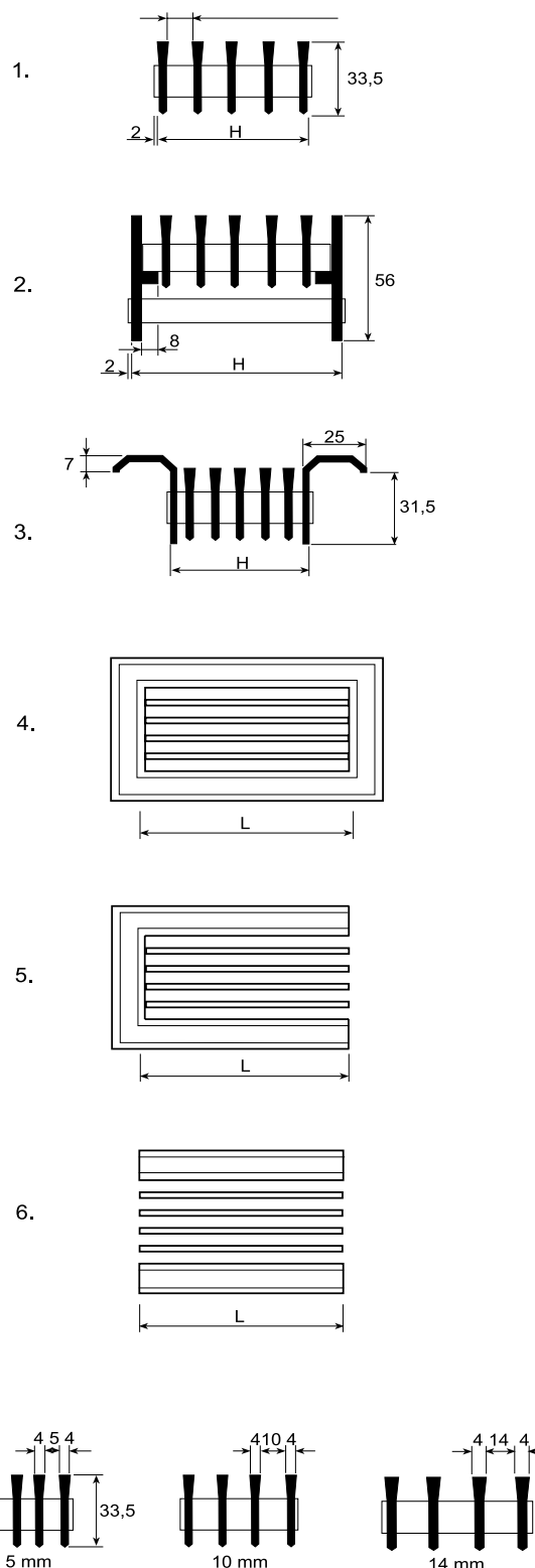
Abbildung 3. Maße.
