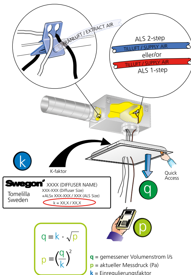
Abbildung 1. Einregulierung
