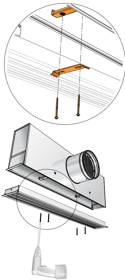
Abbildung 3. Montage von SWAN im SWAN T.
