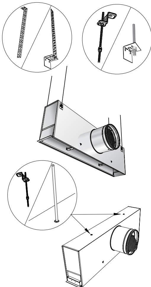
Abbildung 2. Alternative Montage mit Gewindestange, Lochband oder Draht.
