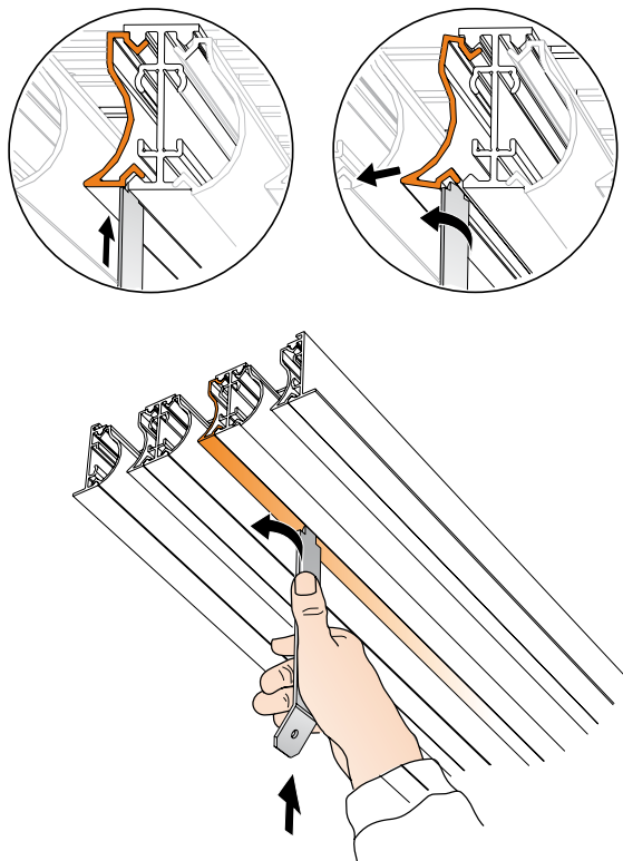
Abbildung 4a. Luftverteiler demontieren.
