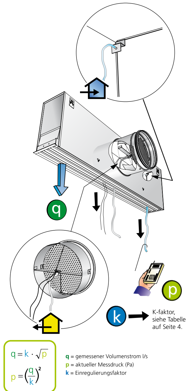
Abbildung 1. Einregulierung und platzierung des Messausgangs.
