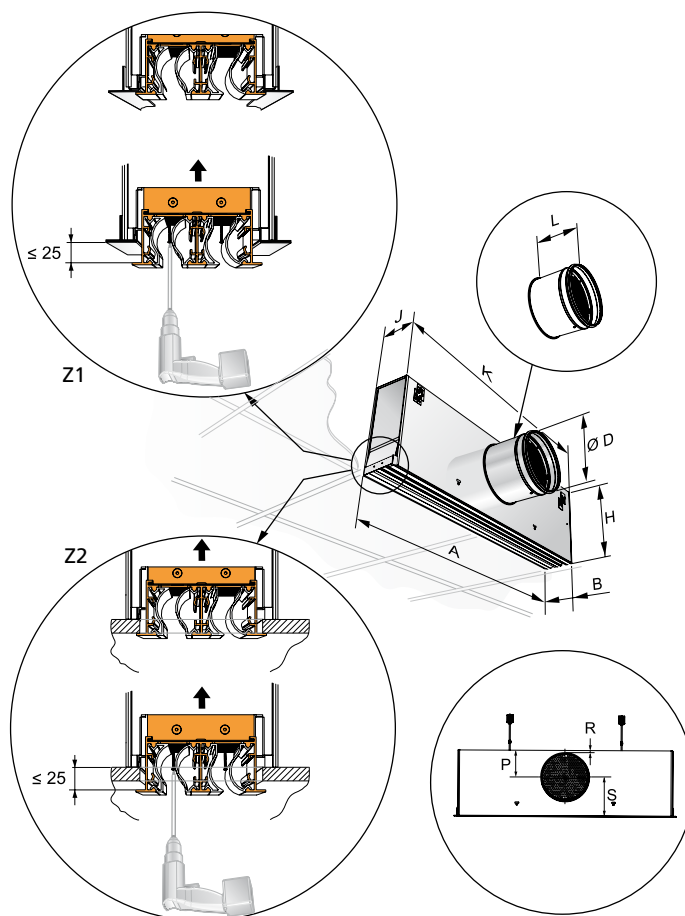
Abbildung 6. SWAN mit Anschlusskasten SWAN T.
