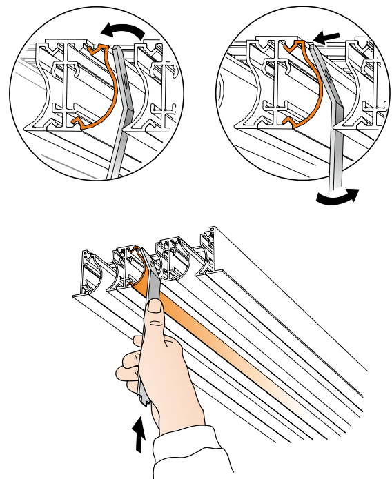
Abbildung 4b. Luftverteiler montieren.
