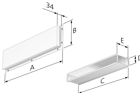
Kuva 2. ROT a , mitat:
